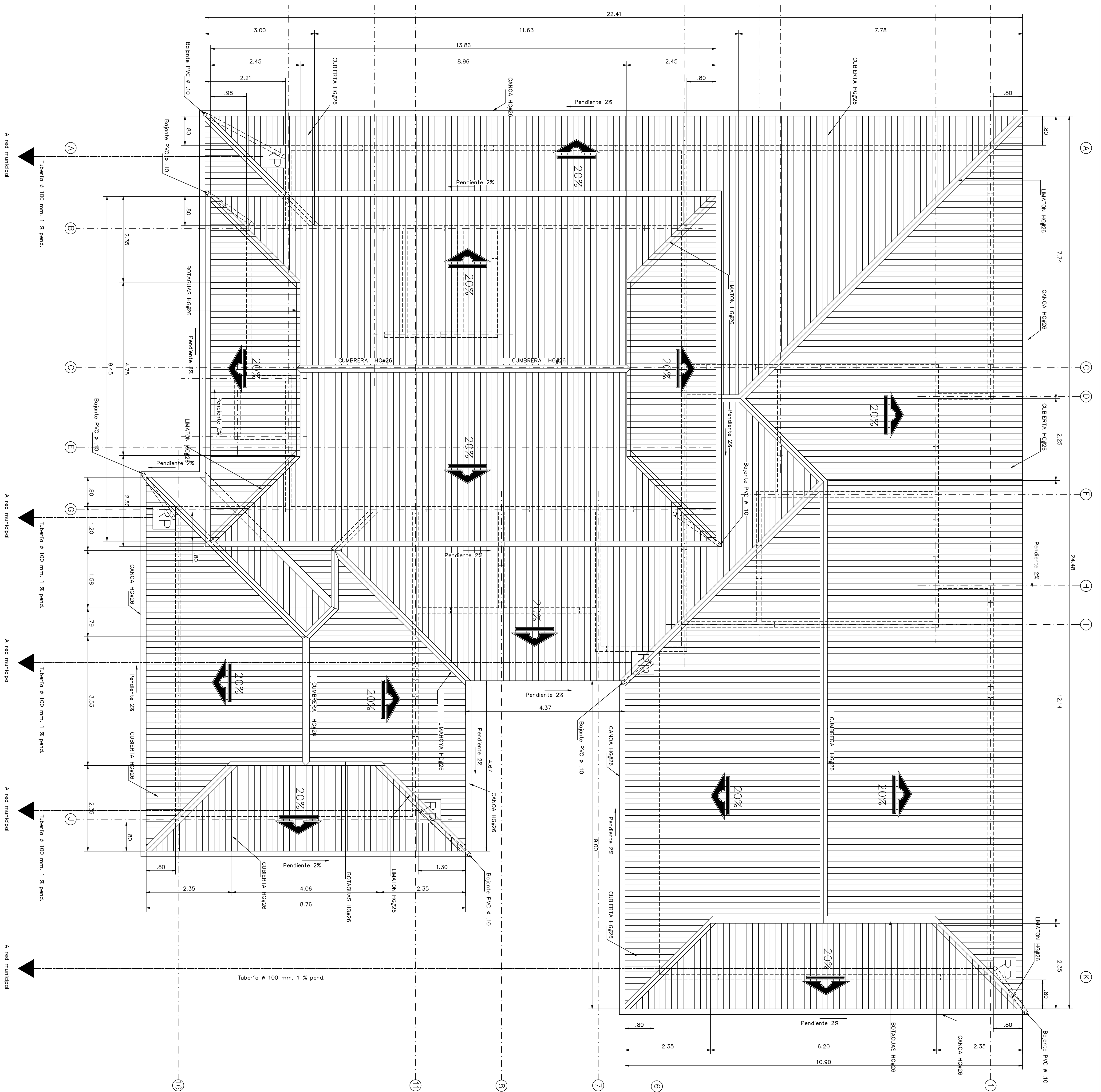
Planta de techos y pluviales Escala 1 : 30
